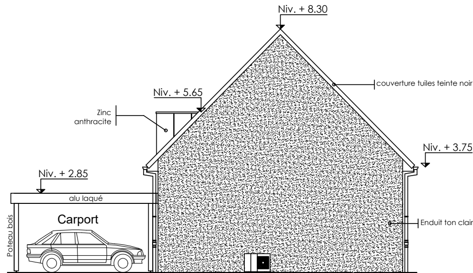
Pignon Droit
